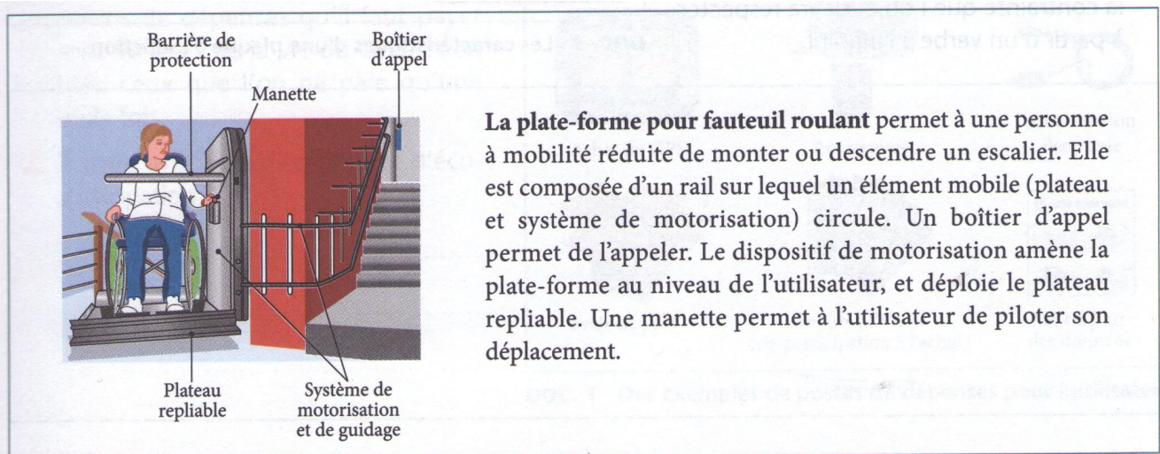
DOC. 1 La structure d'une plate-forme pour fauteuil roulant
